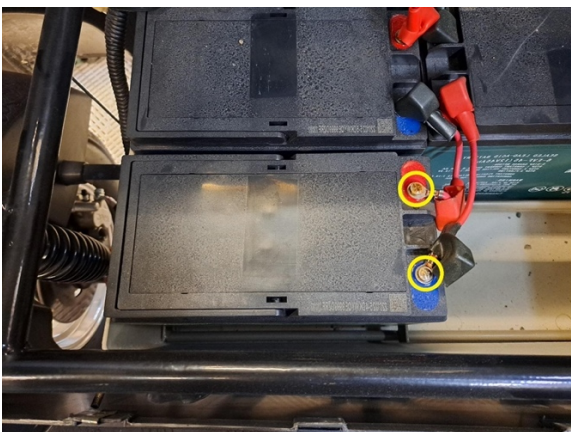
Irrota akun kaapelien kiinnitysruuvit. (ristipäämeisseli ph2). Älä aiheuta oikosulku.
